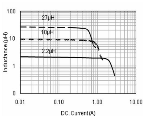
PWPI 3015 TYPE
