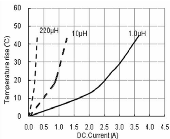
PWPI 4018 TYPE
