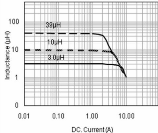
PWPI 8040 TYPE
