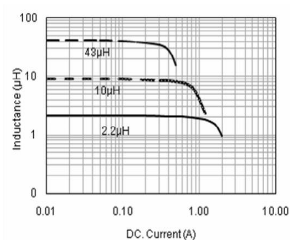
PWPI 3010 TYPE
