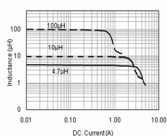
PWPI 4030 TYPE
