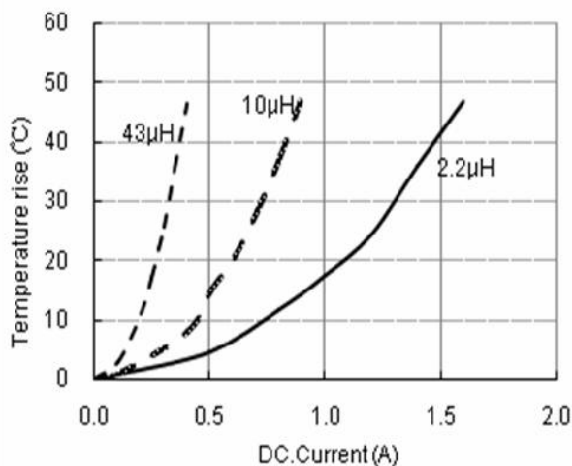
PWPI 3010 TYPE
