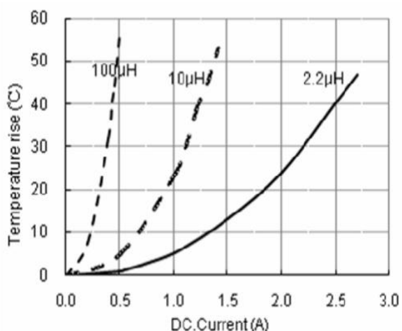
PWPI 4020 TYPE
