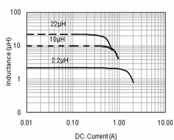
PWPI 4010 TYPE
