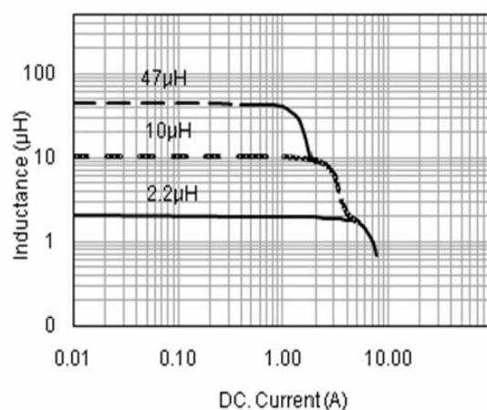
PWPI 6028 TYPE
