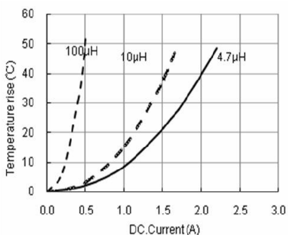
PWPI 4030 TYPE
