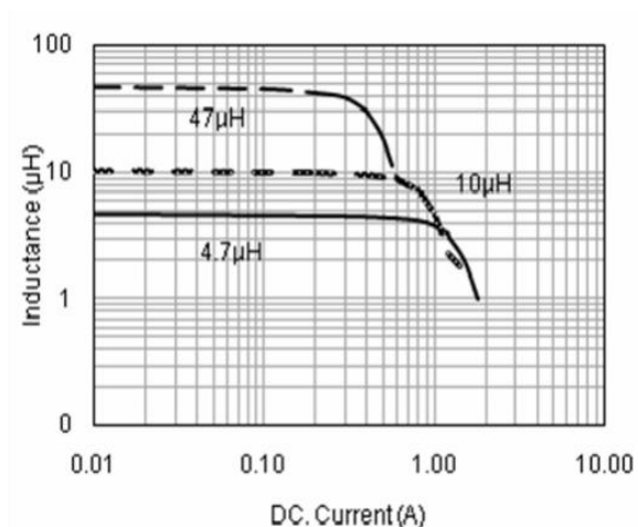
PWPI 3012 TYPE
