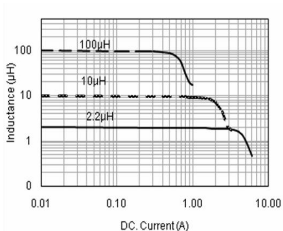
PWPI 4020 TYPE
