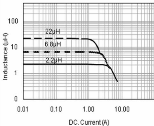
PWPI 6020 TYPE
